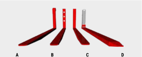
A - FORCHE A PERNO B - FORCHE BULLONATE C - FORCHE SALDATE D - FORCHE TELESOPICHE
