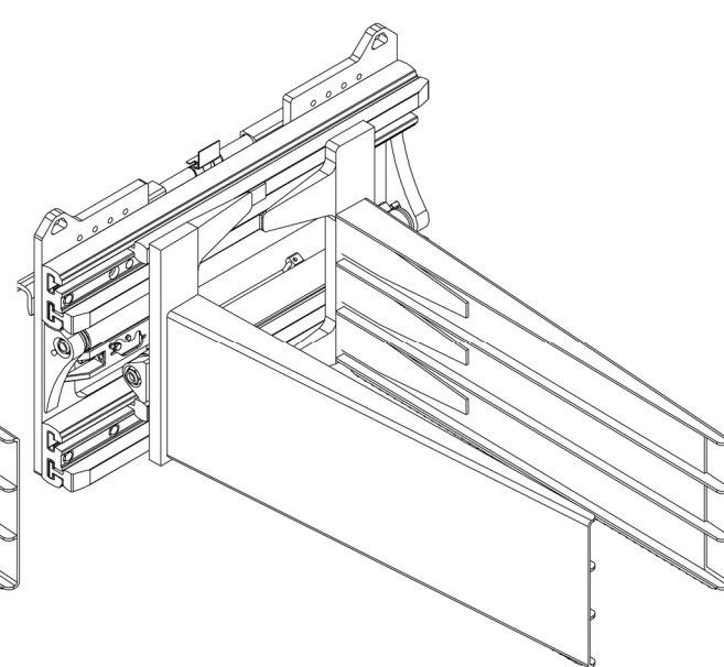
TYPE 474.130 AVEC SLS
