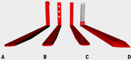
A - FOURCHES PIN-TYPE B - FOURCHES BOULONNÉES C - FOURCHES SOUDÉES D - FOURCHES TÉLESCOPIQUES
