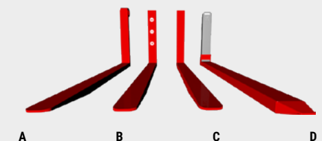
A - WELLENGABELN B - ANGESCHRAUBTE GABELN C - ANGESCHWEISSTE GABELN D - TELESKOPGABELN
